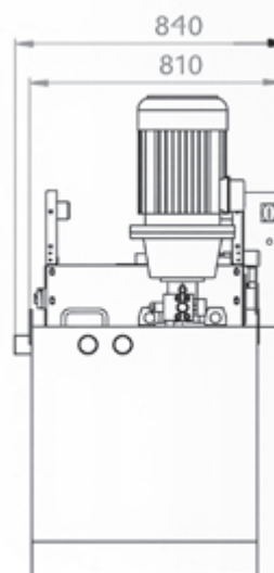
PLUS-järjestelmän päämitat
