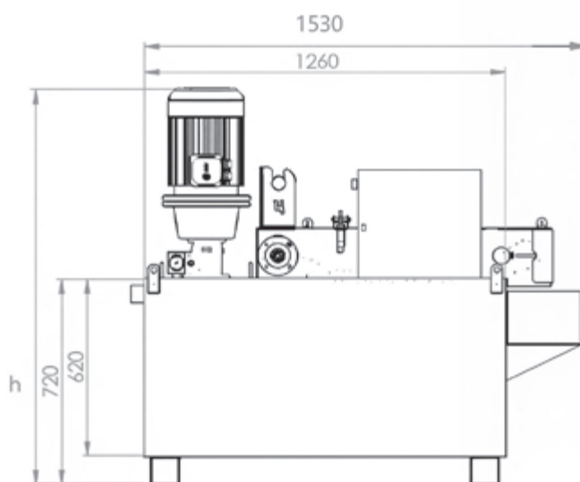
PLUS-järjestelmän päämitat
